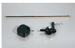
Figur 1: Dobbelt brænderudstyr
